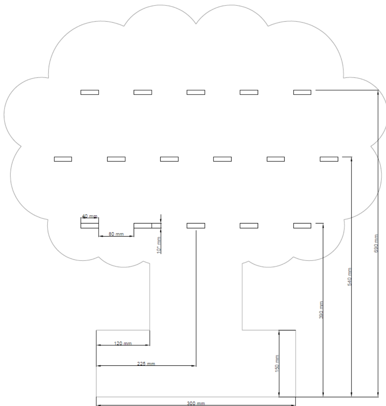
Figura 9. Dimensiones del árbol
