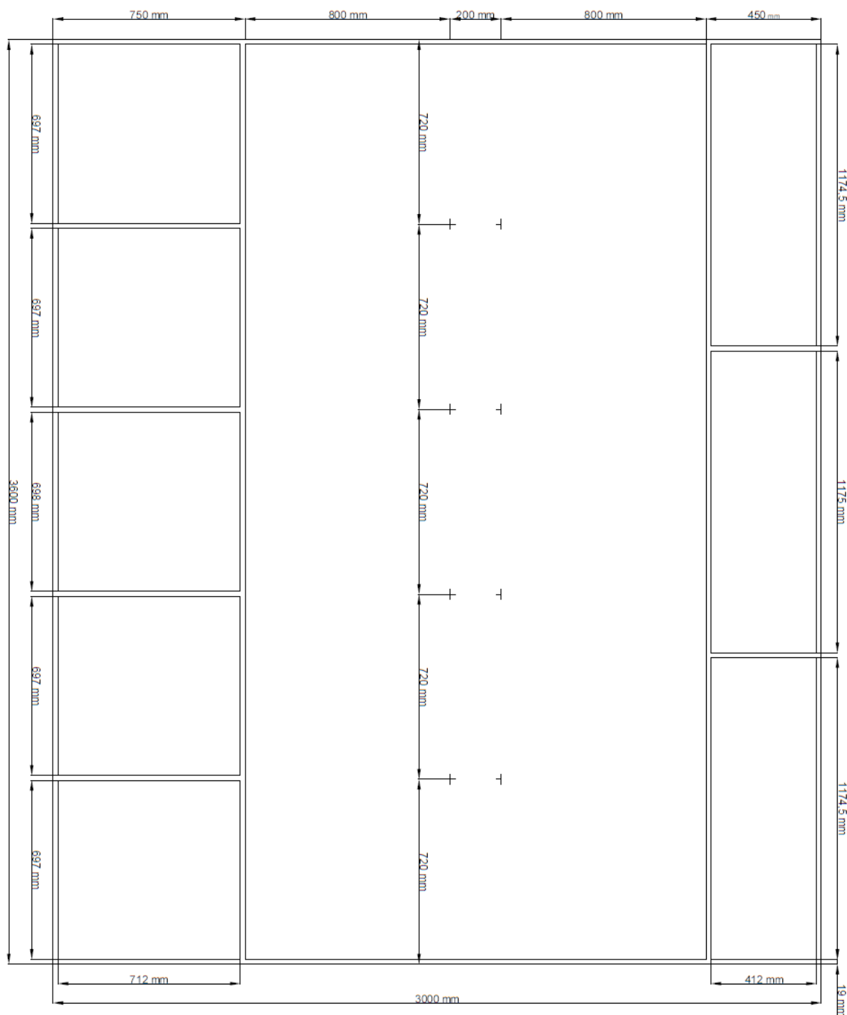
Figura 8. Dimensiones del escenario
