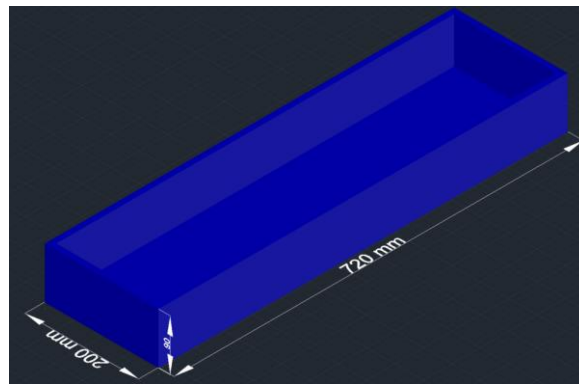
Figura 7. Dimensiones de la alberca.
